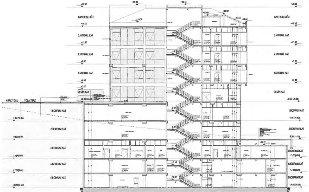
2-2 KESİTİ ÖLÇEK :1/100
