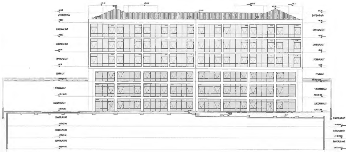
GÜNEY CEPHESİ ÖLÇEK : 1/100
