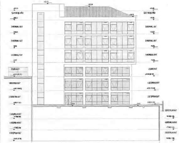
BATI CEPHESİ ÖLÇEK :1/100
